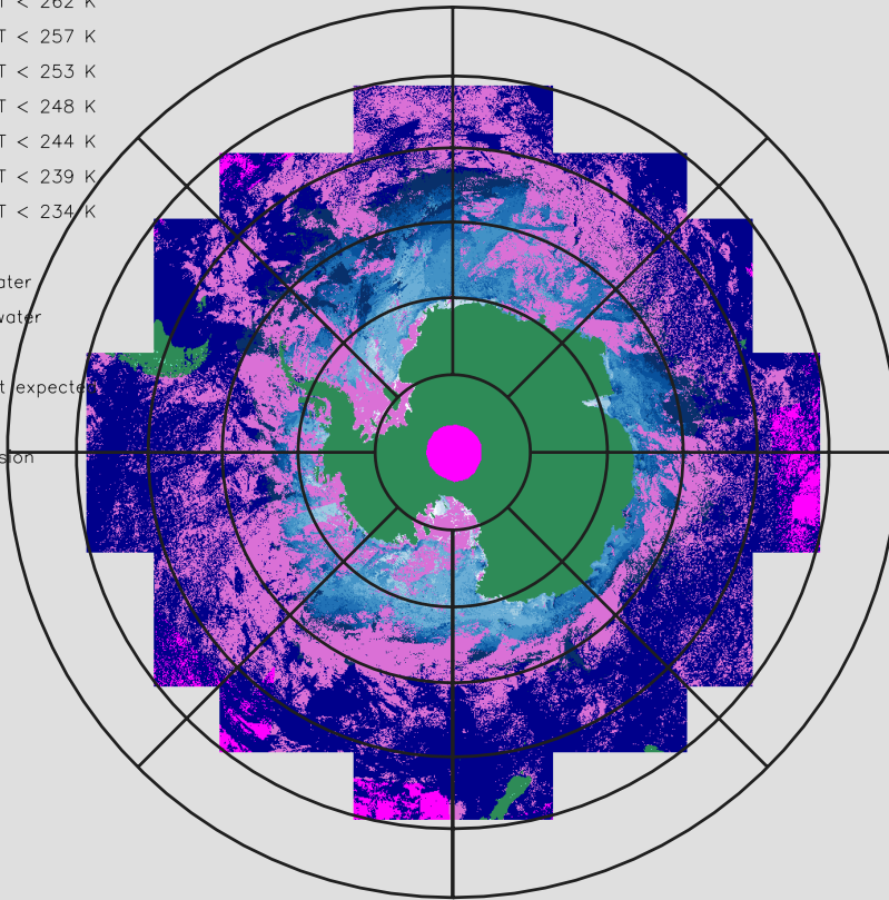
MYD29E1D.A2003258 9-day Composite IST
